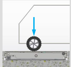
Überfahrbarkeit , mit 6 t Radlast
